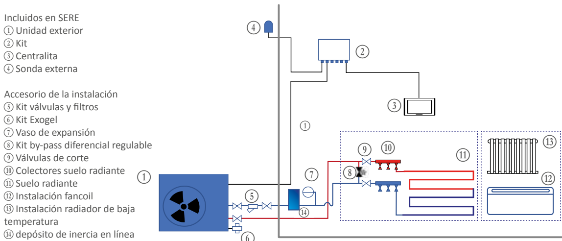
Gráfico 4-15. Caso tipo 2. Piso en bloque. Opción 100% hidráulica. Esquema de principio universal para calefacción con tres tipos de emisores posibles: suelo radiante, fancoils o radiadores de baja temperatura
