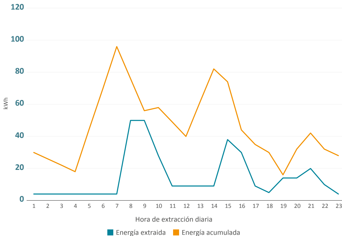
Gráfico 4-44. Caso tipo 5. Centralizada. BdC de producción instantánea de ACS. bomba de calor ON-OFF y producción
