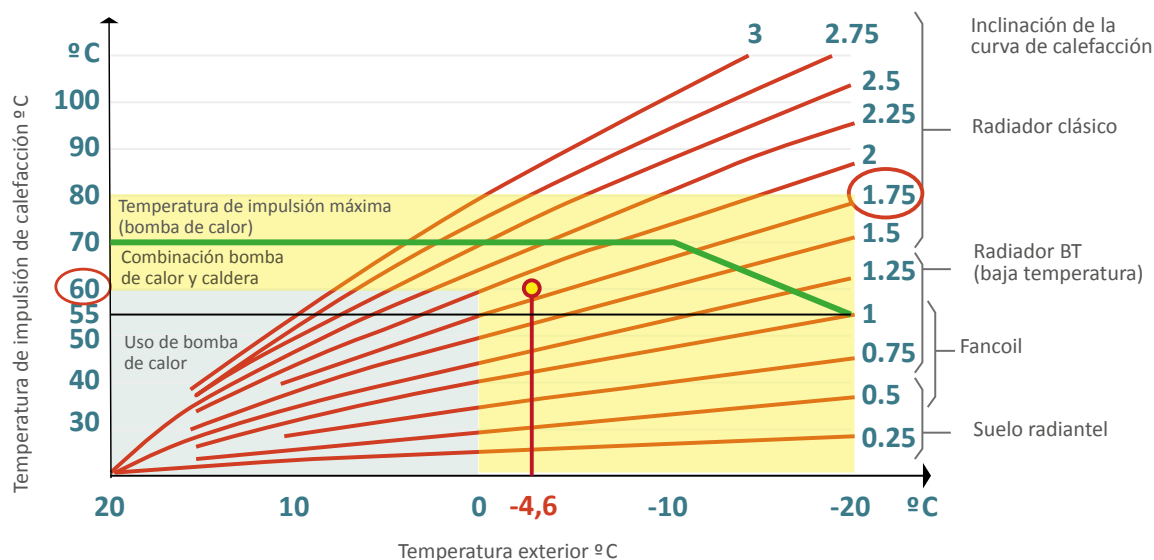
Gráfico 4-37. Caso tipo 4. Curva seleccionada para el funcionamiento en régimen de 24 horas, durante la temporada de calefacción
