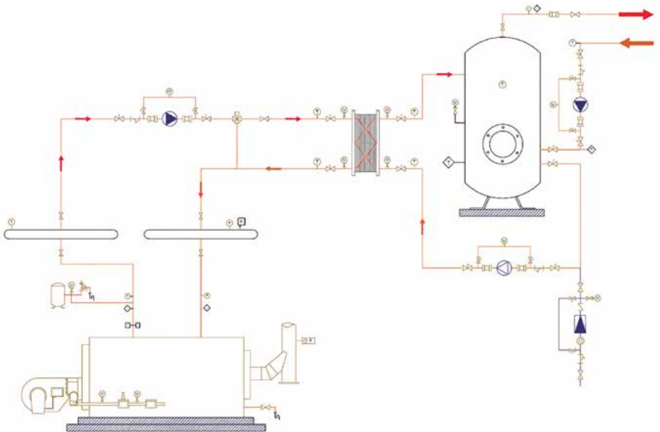
Gráfico 4-43. Caso tipo 5. Centralizada. Bomba de calor de producción instantánea de ACS. Esquema de la instalación existente
