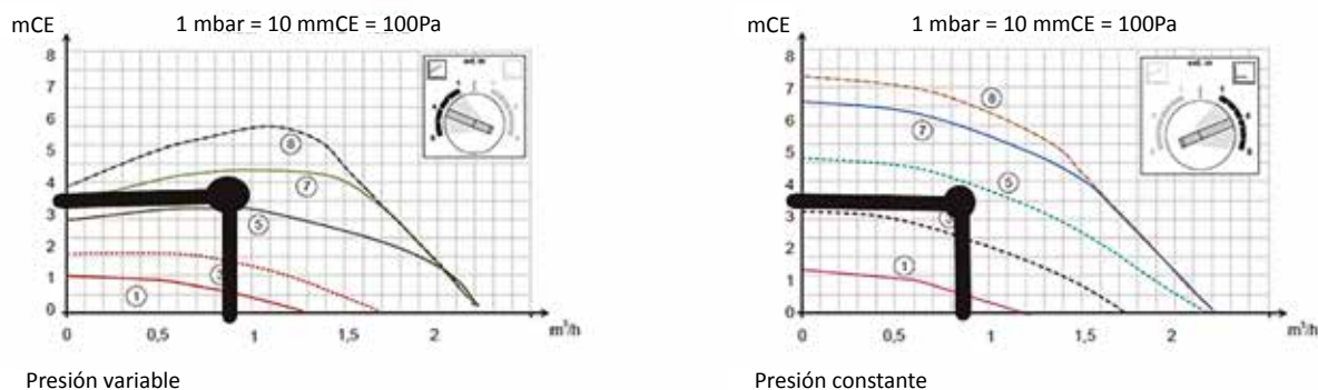
Gráfico 4-9. Caso tipo 1. Vivienda unifamiliar. Gráfico de línea de pérdida de carga de la instalación vs. presión disponible y caudal en bomba circuladora
