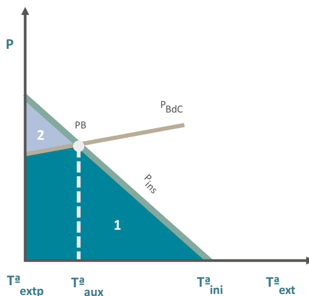
Gráfico 2-63. Sistema bivalente paralelo
