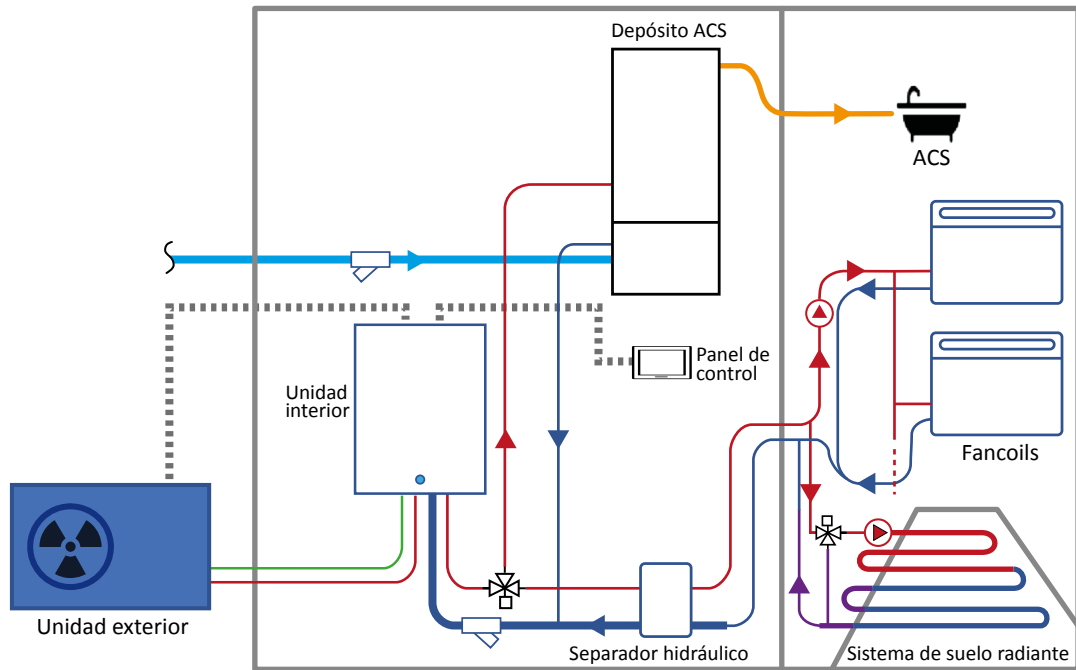
Gráfico 2-31. Ejemplo de sistema con bomba de calor para tres servicios, ACS, S. Rad. y fancoils
