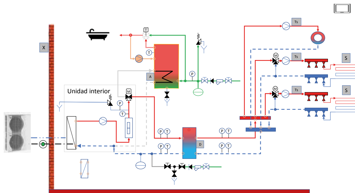
Gráfico 5-2. Caso de éxito uno. Esquema de principio
