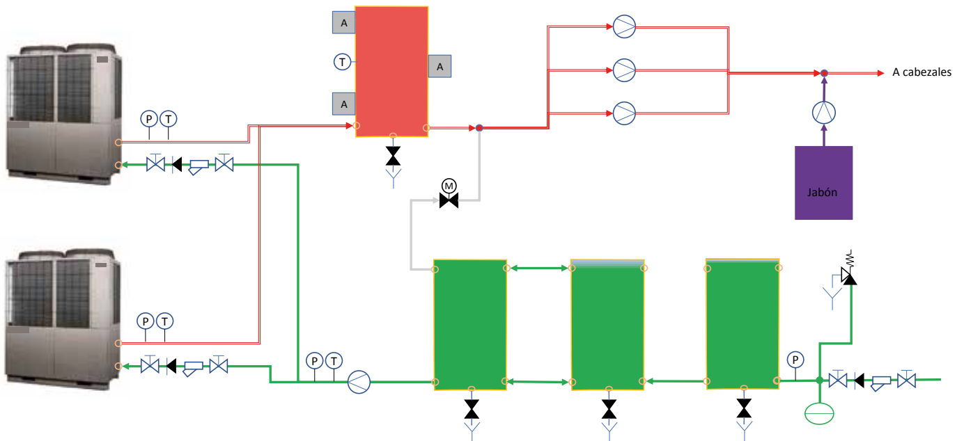
Gráfico 5-28. Caso de éxito once. Esquema de principio
